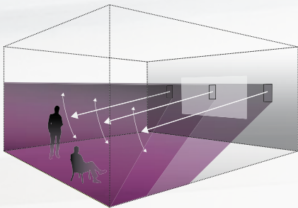
DE Plan 600 AIArray , Wandeinbau mit einstellbarem Abstrahlwinkel
