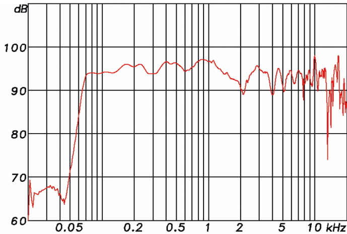
F 12 hor. Direktivität Plot
