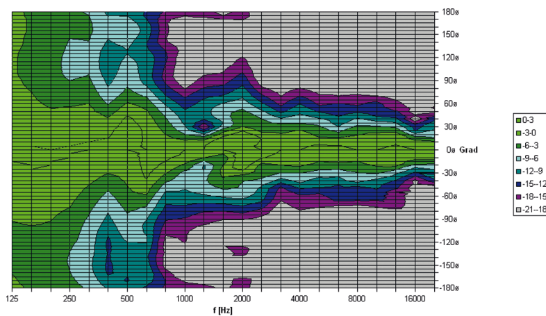
F 12 vert. Direktivität Plot
