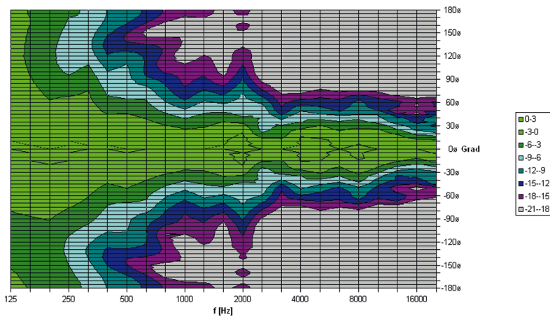
F 12 hor. Direktivität Plot
