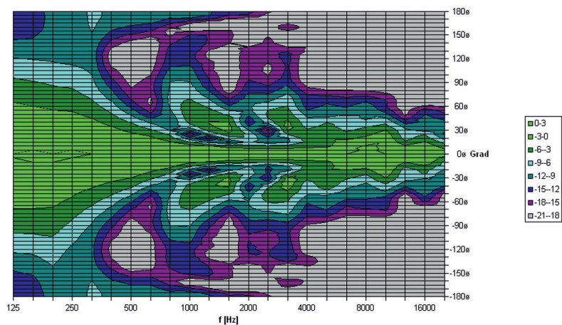
RL 206 SN vert. Direktivity Plot
