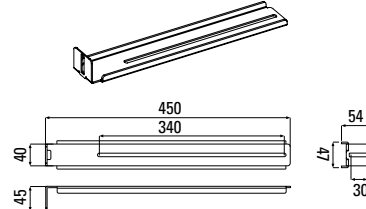
DL-VESA L-Bracket 450 mm for DL-VESA 2000 ... 2600
